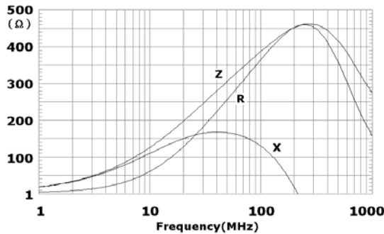
EBMS160808A401
