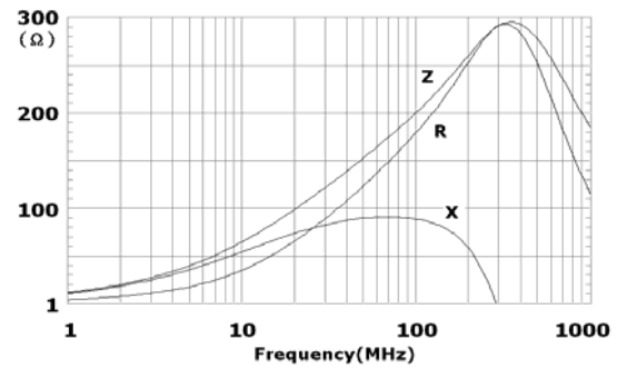
EBMS160808A301
