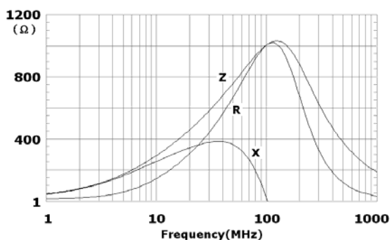
EBMS160808B050
