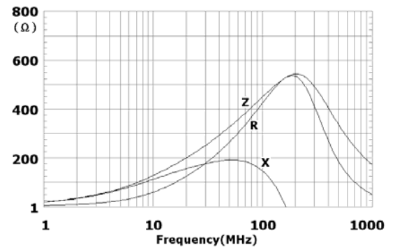
EBMS160808A451
