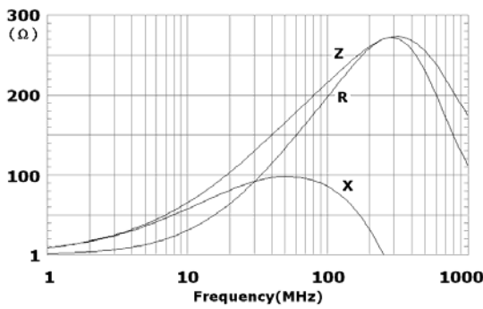
EBMS160808A401
