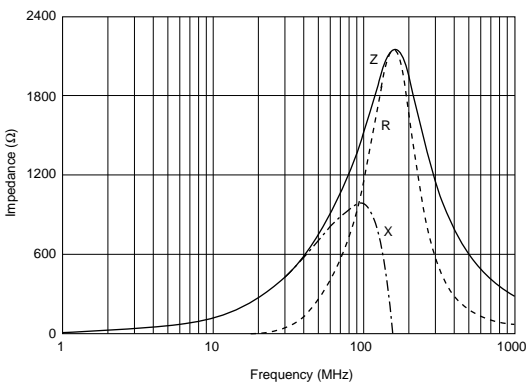
BLM21BD152SN1
