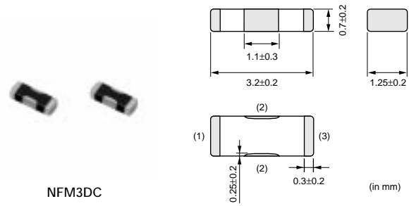
NFM3DC
